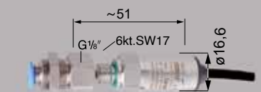
Flüssigkeitsdrucksensor
